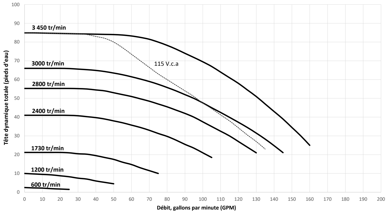
Courbes de performance VSSH270DV2A
