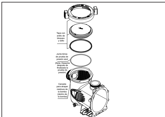
Figura 14. Vista ampliada con junta tórica de prueba de presión azul (modelos de bomba VSSHP únicamente)
