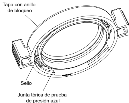
Figura 13. Junta tórica de prueba de presión azul
