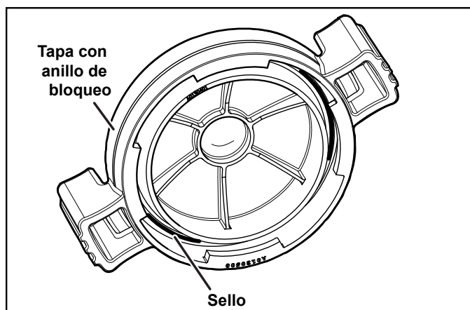
Figura 17. Junta tórica en el conjunto de la tapa
