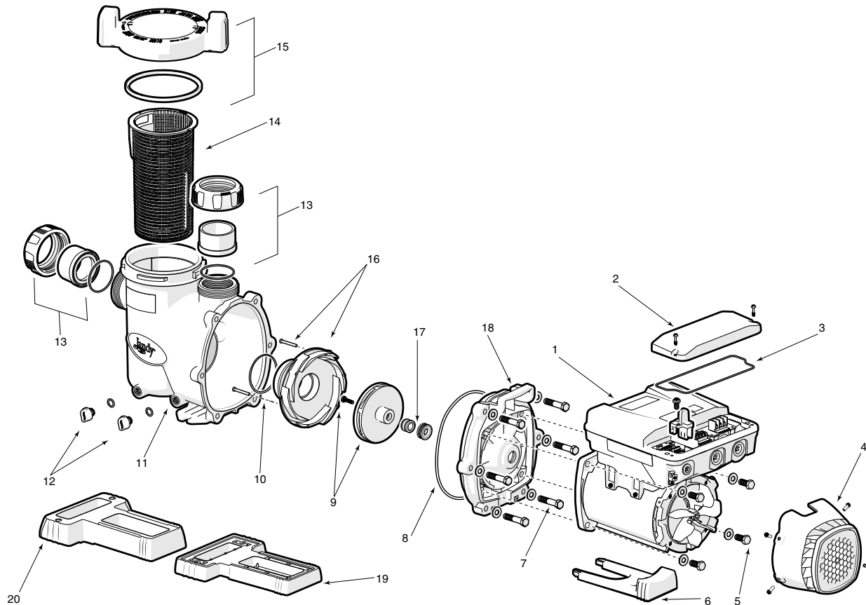
Figura 19. Vista ampliada de la bomba de velocidad variable modelo Jandy DV2A
