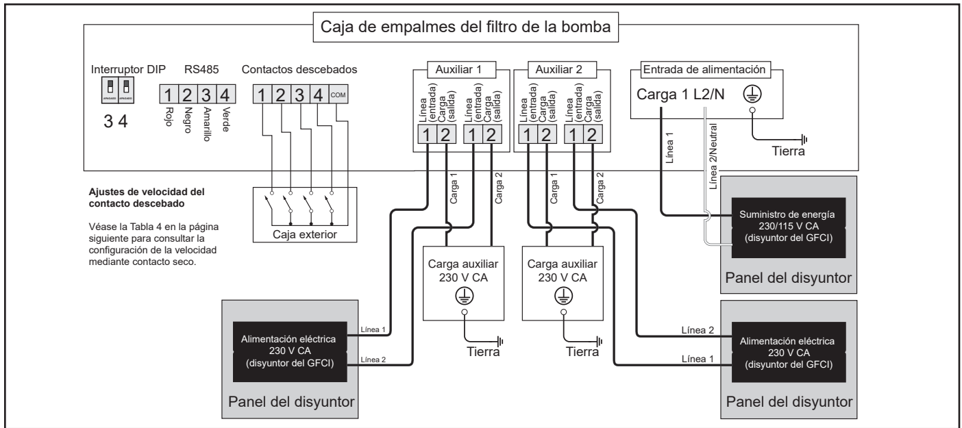
Figura 10. Diagrama de cableado de relé auxiliar de 230 V*
