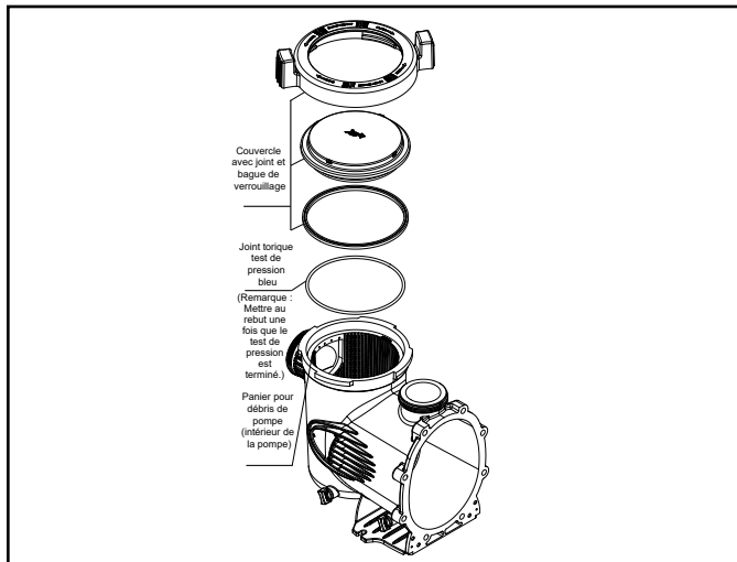
Figure 14. Vue éclatée avec le Joint torique test de pression bleu (Modèles de pompe VSSHP uniquement)
