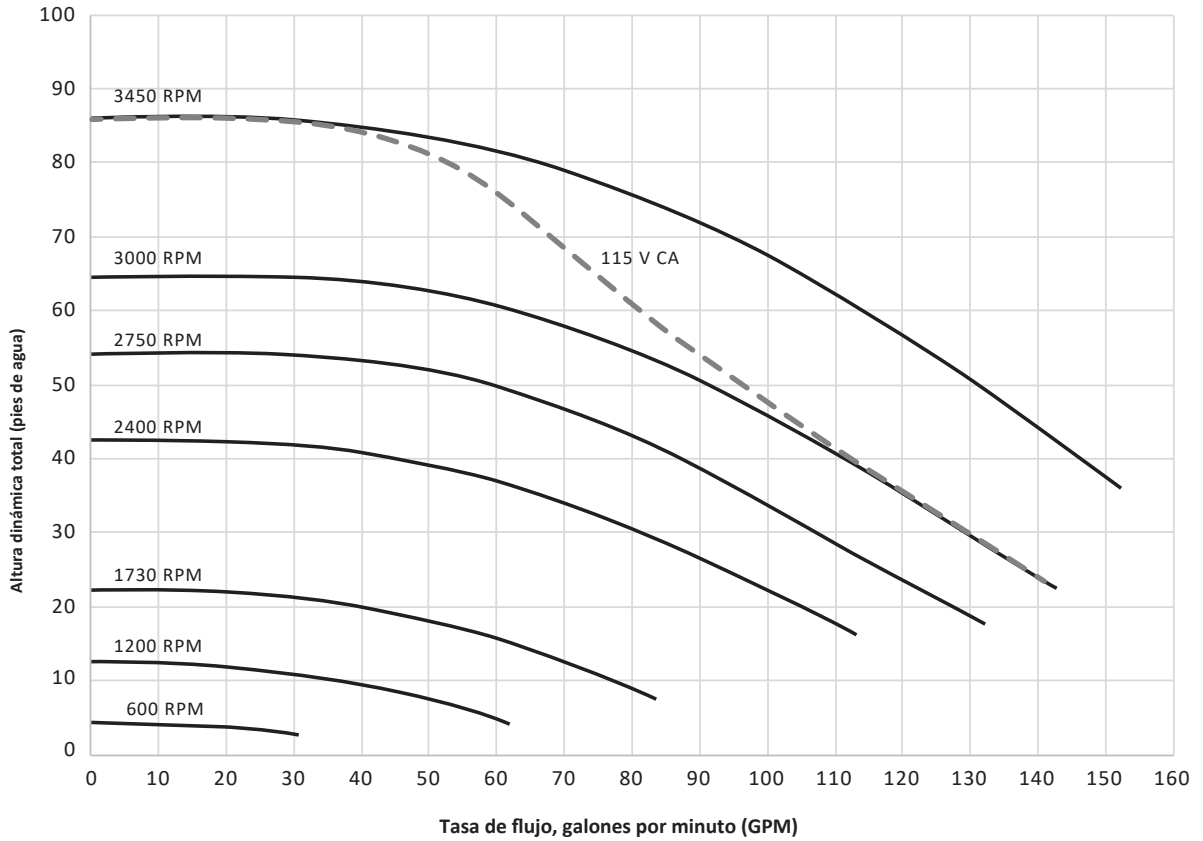
Curvas de desempeño VSPHP270DV2A
