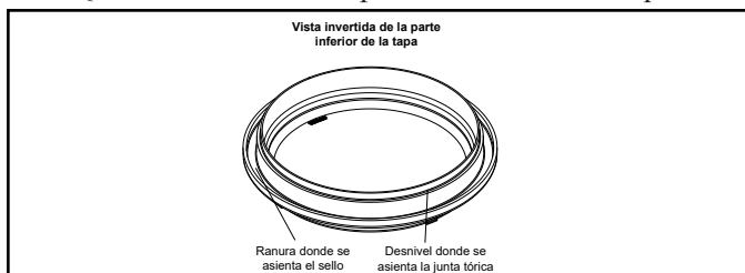
Figura 15. Colocación de la junta tórica de prueba de presión azul
