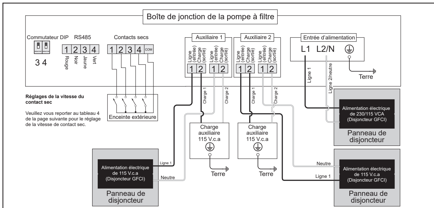
Figure 11. Schéma de câblage du relais auxiliaire de 115V*
