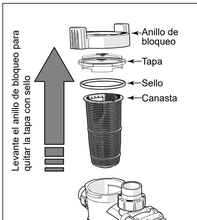
Figura 18. Quitar la tapa de la bomba
