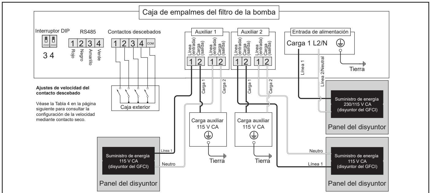
Figura 11. Diagrama de cableado de relé auxiliar de 115V*
