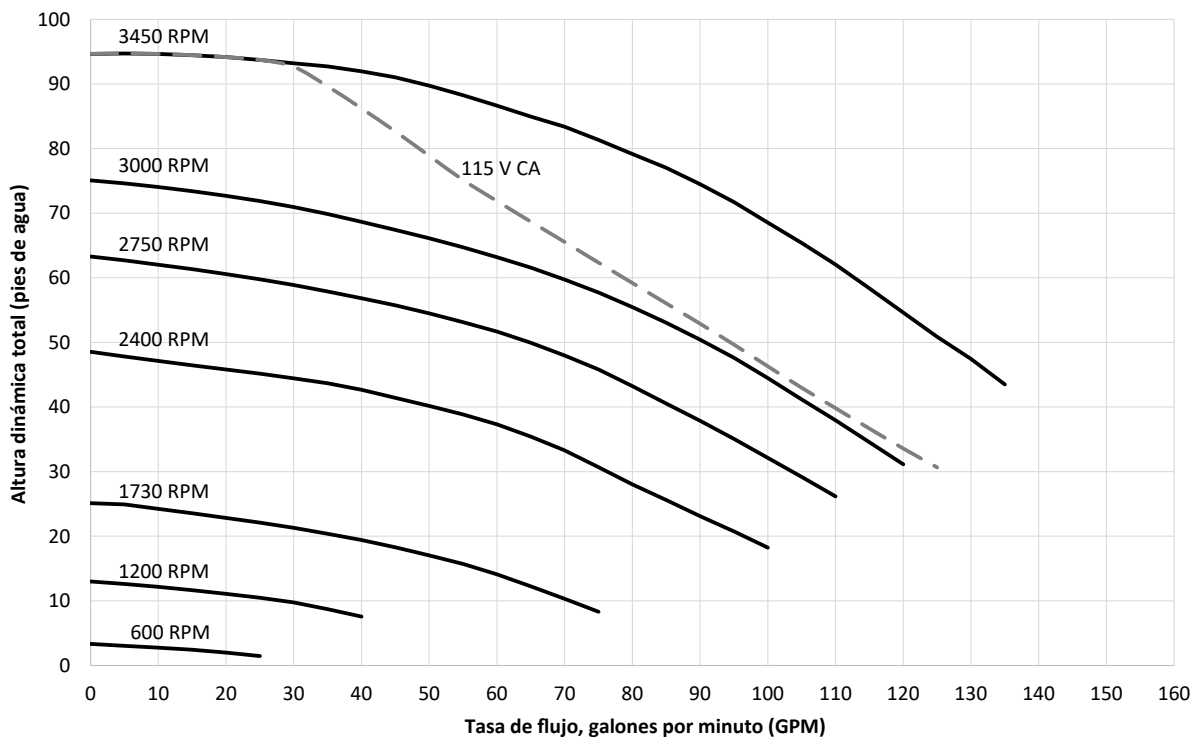
Curvas de desempeño VSFHP270DV2A
