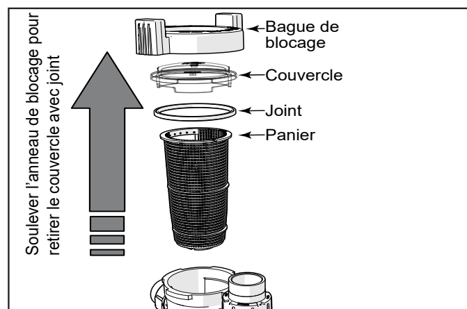
Figure 18. Retirer le couvercle de la pompe
